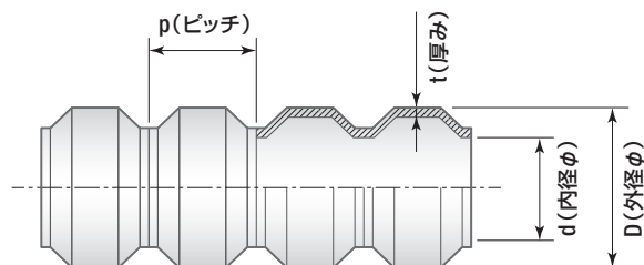
※1. コルゲートチューブ 製品寸法図
