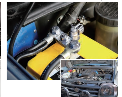
スズキジムニー JB23(SUZUKI Jimny JB23)
