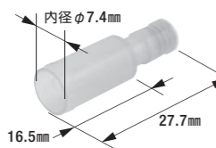
A-201B 防水型絶縁被覆付ピンターミナル
