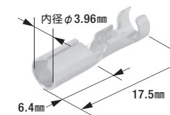
B-2-24K ギボシ端子(24K(金メッキ)仕様)
