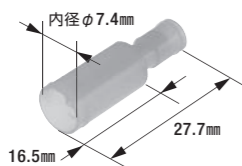
A-101 絶縁被覆付ピンターミナル
