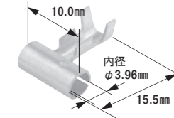
B-31 ギボシ端子(L形)
