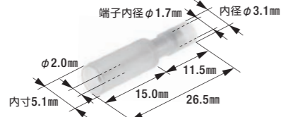
A-001 絶縁被覆付ピンターミナル
