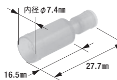
A-201 防水型絶縁被覆付ピンターミナル
