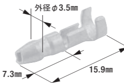
B-41 ギボシ端子(小)
