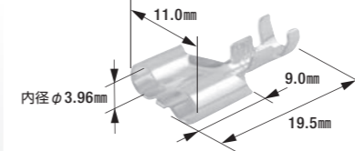
B-16 ギボシ端子(W形)
