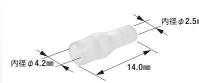
B-3 絶縁スリーブ
