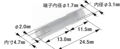
A-002 絶縁被覆付ピンターミナル
