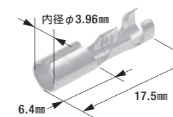
B-2 ギボシ端子
