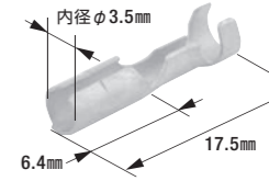
B-42 ギボシ端子(小)
