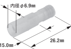
A-202B 防水型絶縁被覆付ピンターミナル
