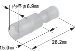
A-202 防水型絶縁被覆付ピンターミナル
